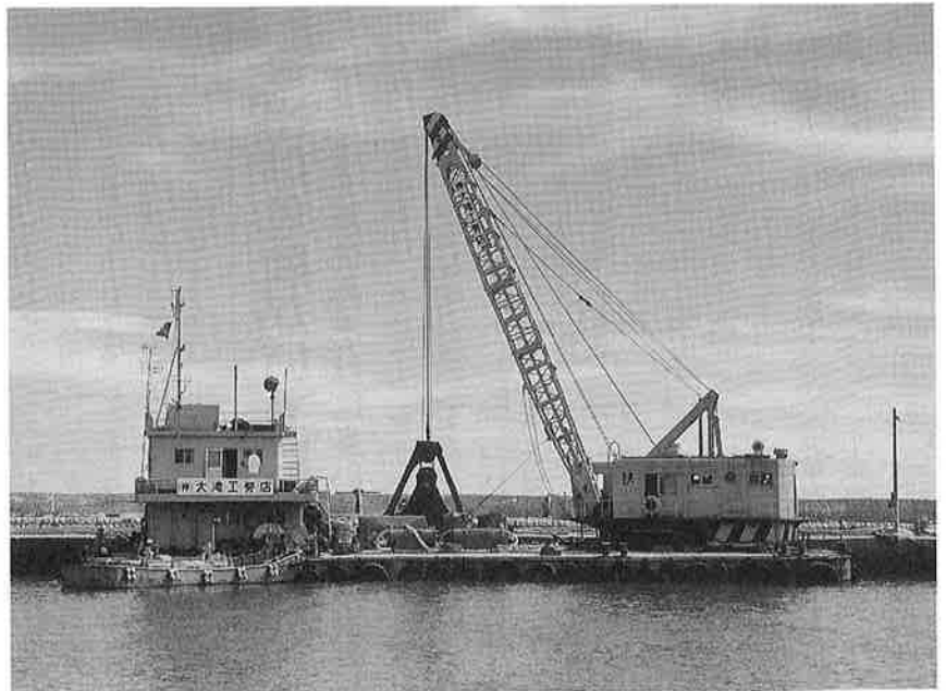
岩和田港に着船中の浮泥除去作業船
